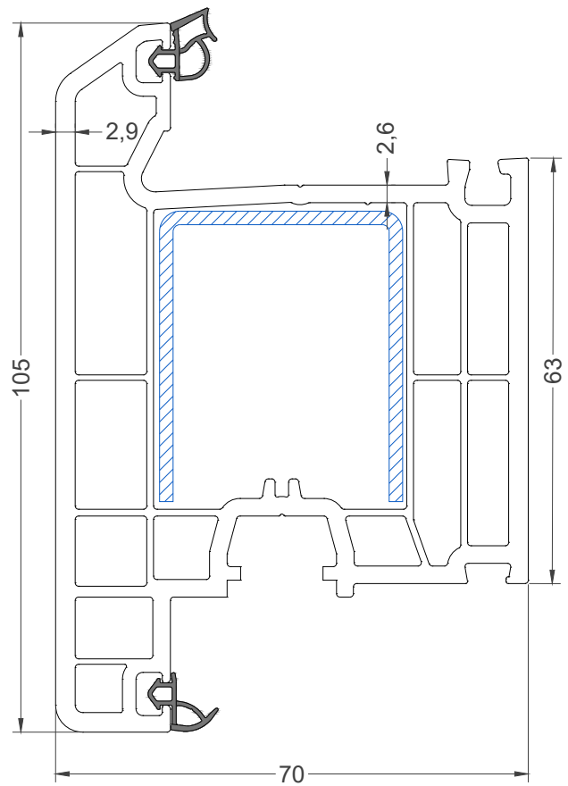
Дверная створка 105 мм (T-type) Арт. 7005
