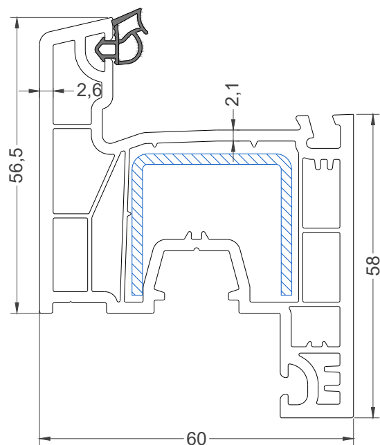
Створка 56.5 мм Арт. 6102
