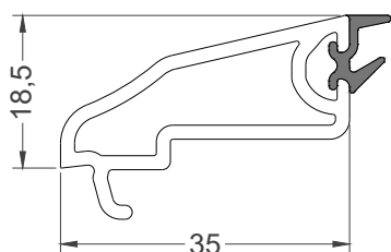
Штапик 4 мм Арт. 6014
