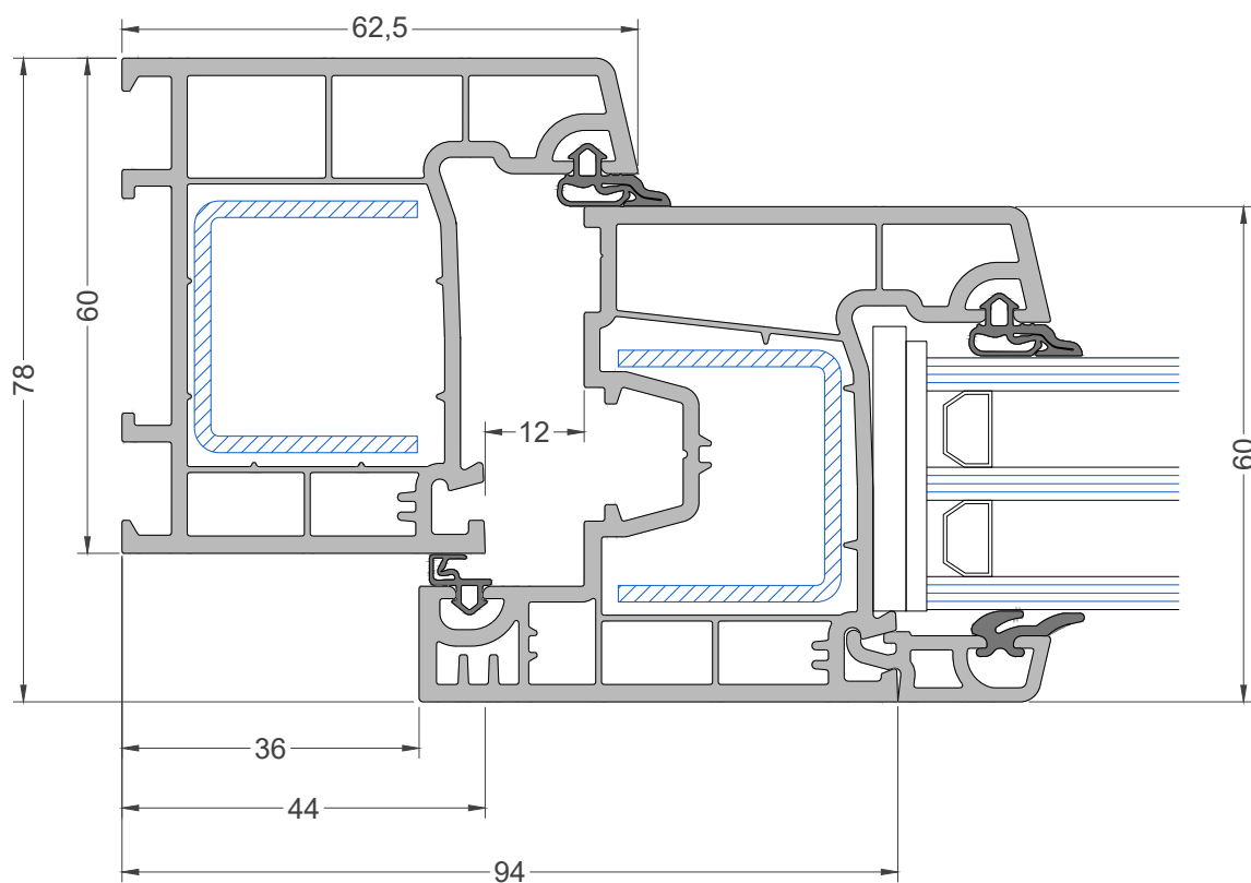
Рама Арт. 6001
