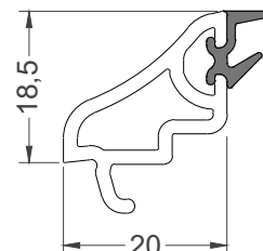
Штапик 20 мм Арт. 6015
