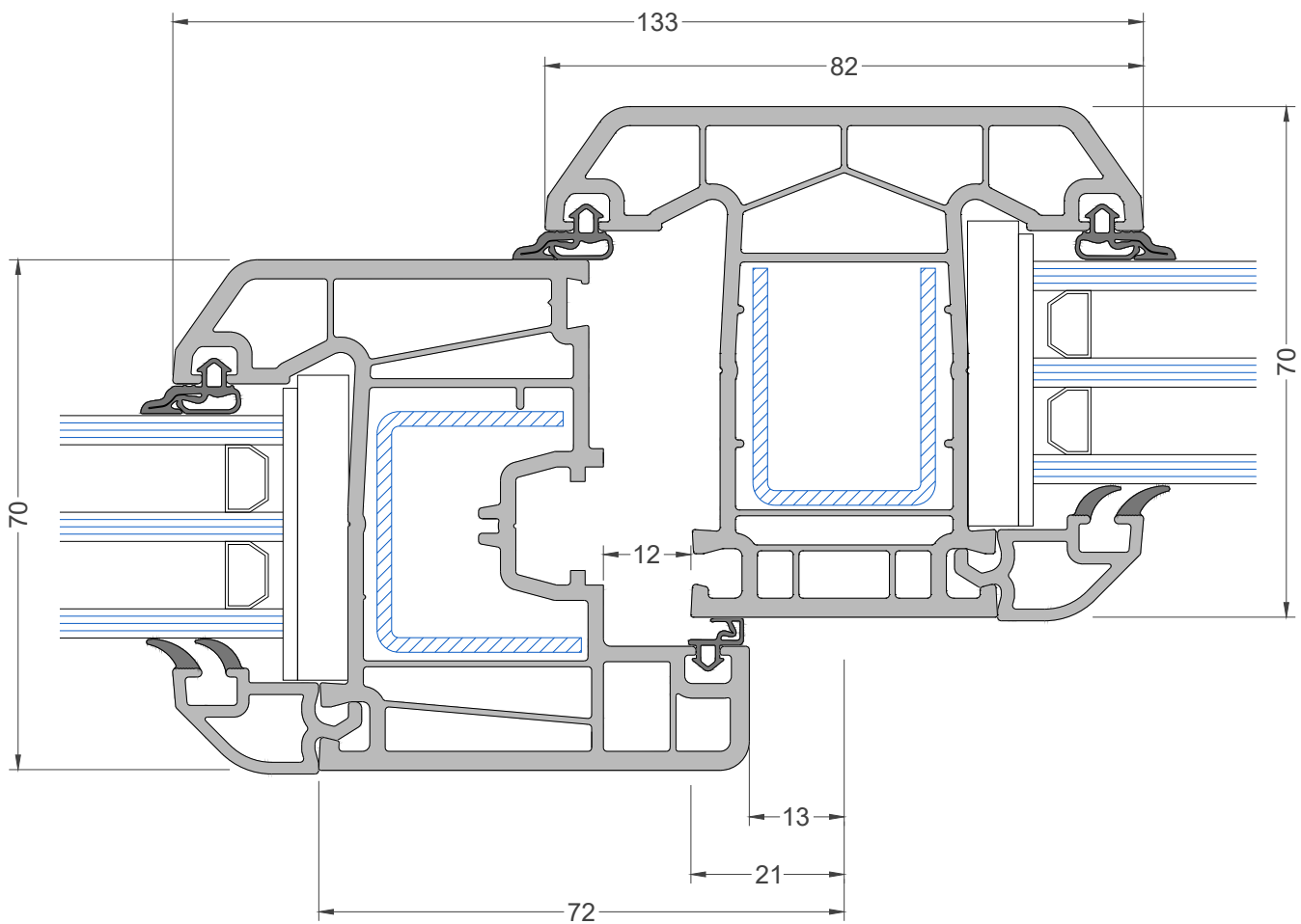
Створка 56.5 мм Арт. 7002
