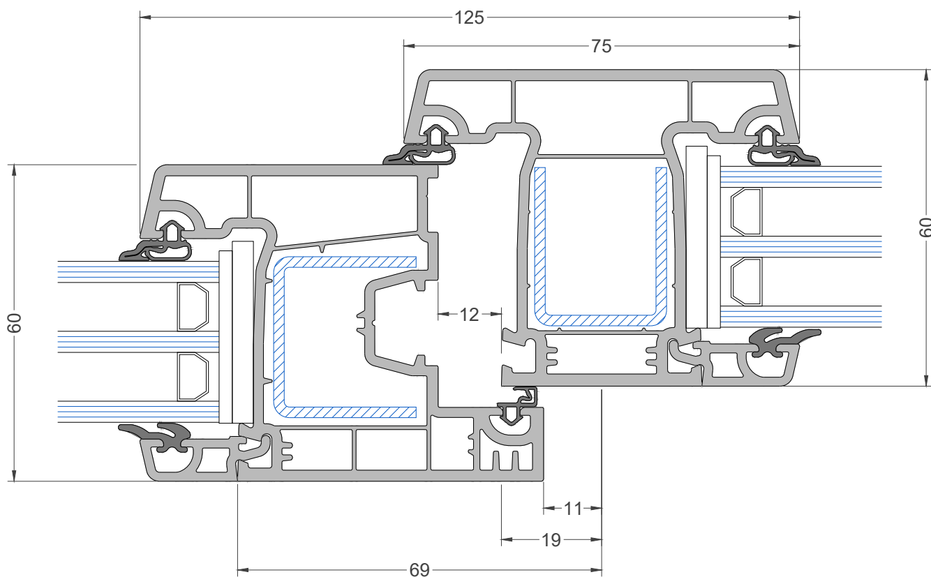
Створка Арт. 6002
