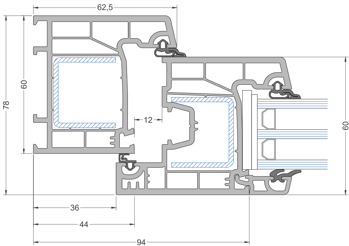
Арт. 6101 Рама
