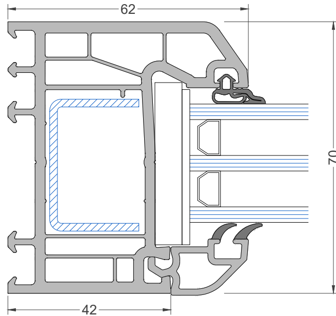
Рама 62.5 мм Арт. 7101
