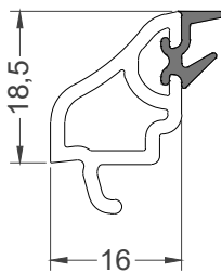
Штапик 24 мм Арт. 6016
