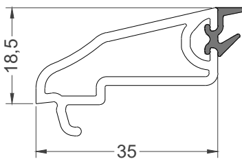
Штапик 4 мм Арт. 6014
