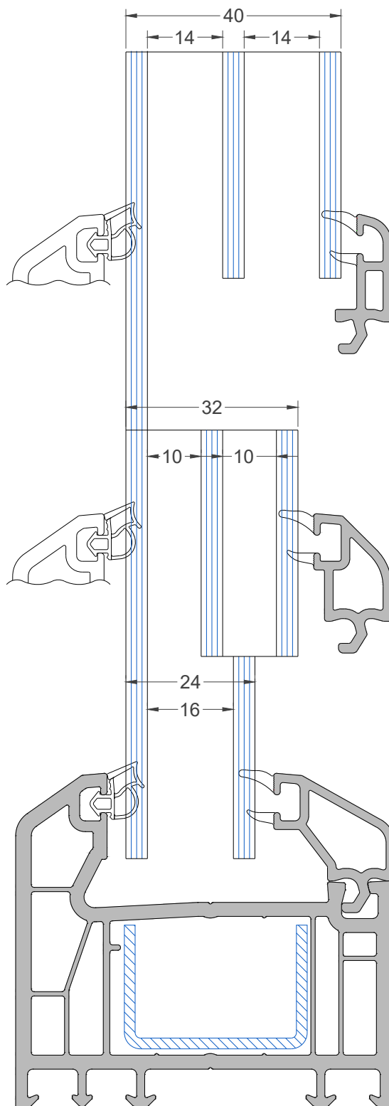
Штапик 40 мм Арт. 7012
