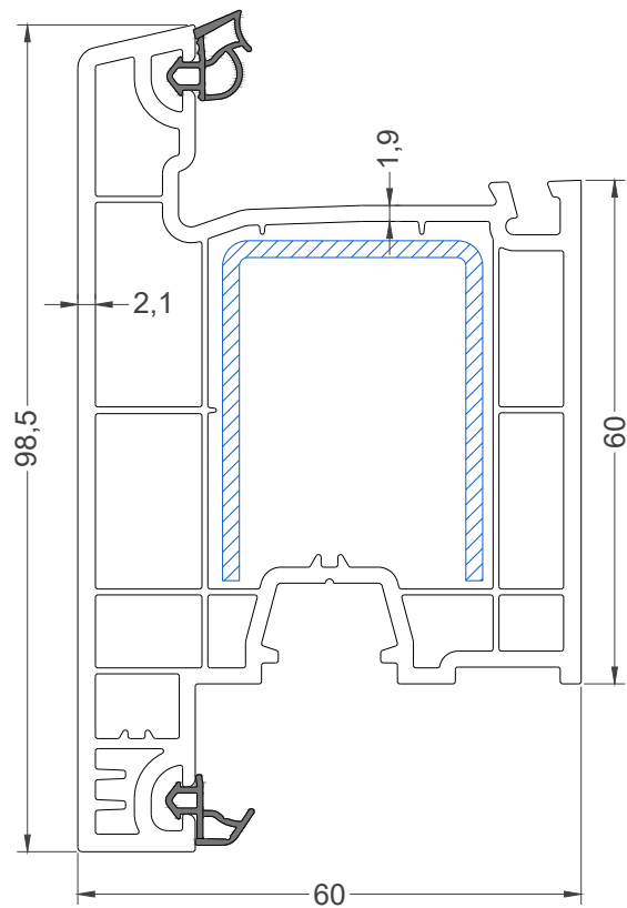
Дверная створка 98.5 мм (T-type) Арт. 6005
