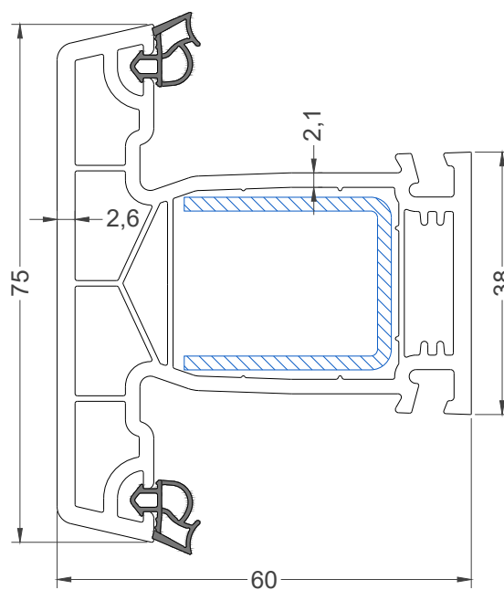
Импост 75 мм Арт. 6103
