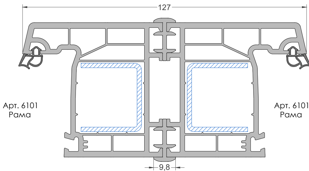
Соединитель рамный Арт. 6012
