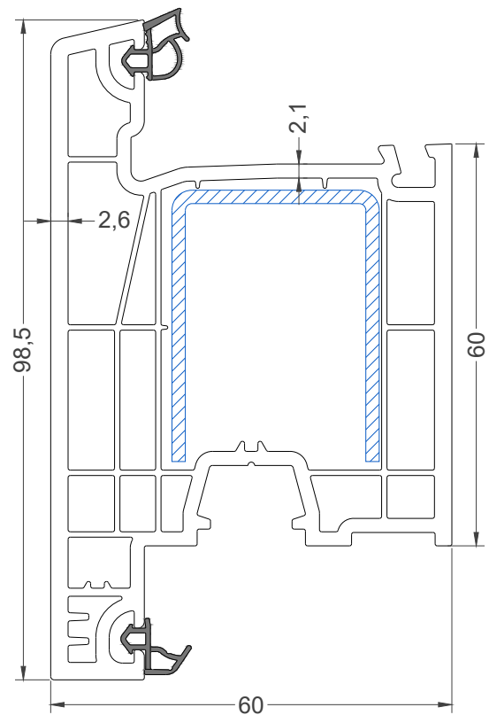
Дверная створка 98.5 мм (T-type) Арт. 6105
