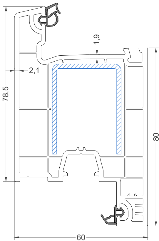
Дверная створка 78.5 мм (Z-type) Арт. 6004
