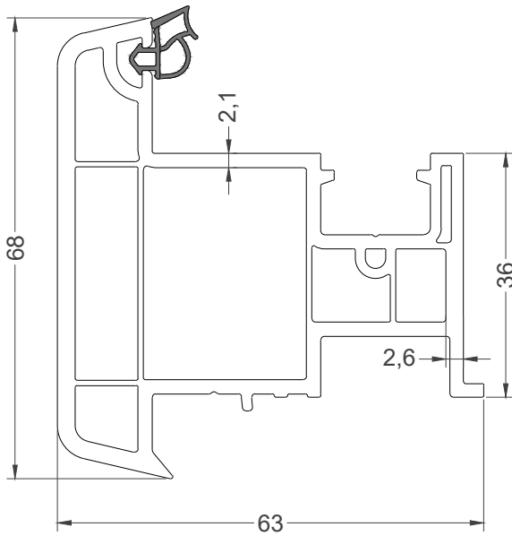
Штульп Арт. 6009
