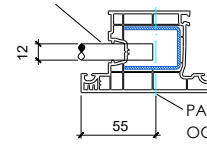
ОТВЕРСТИЕ ШПИНГАЛЕТА 12 мм
