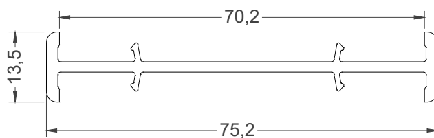
Соединитель рамный 13,5 мм Арт. 7011
