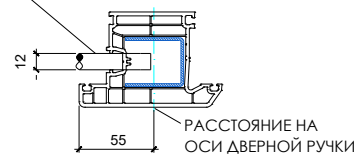
ОТВЕРСТИЕ ШПИНГАЛЕТА 12 мм
