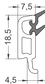
Штапик 20 мм Арт. 6015
