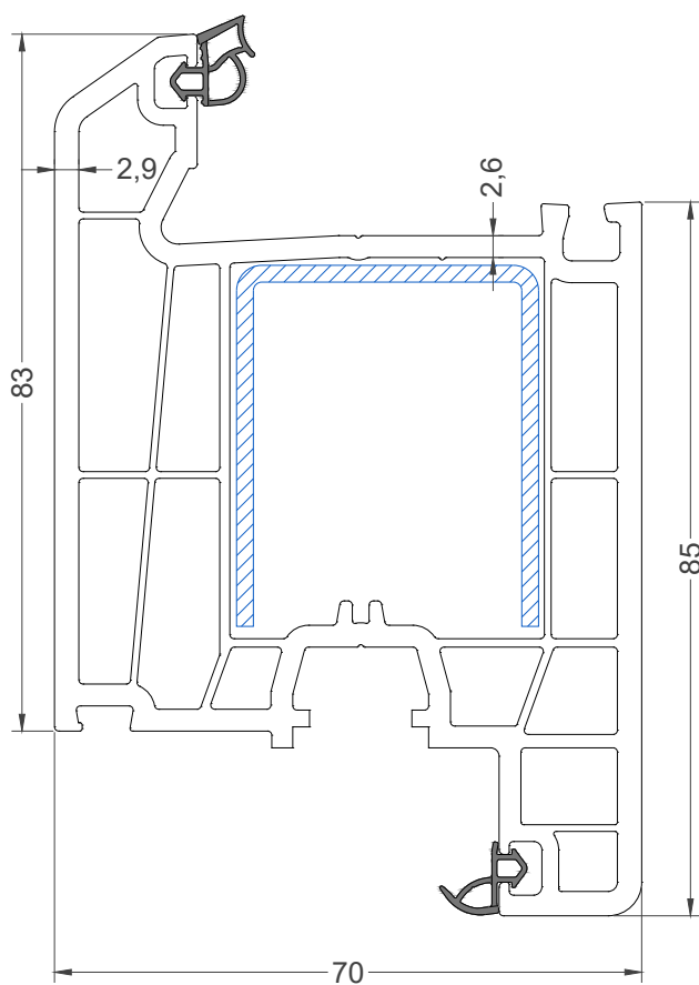
Дверная створка 83 мм (Z-type) Арт. 7004
