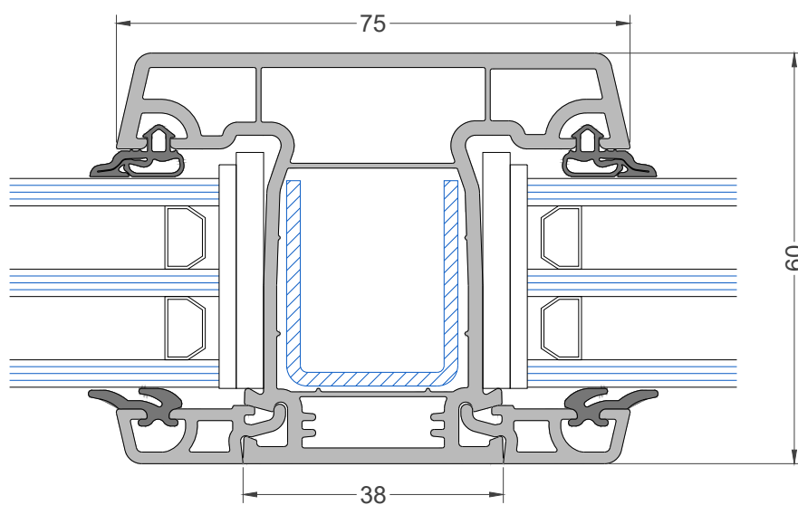
Импост Арт. 6003
