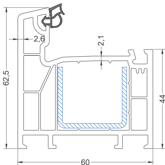
Рама 62.5 мм Арт. 6101
