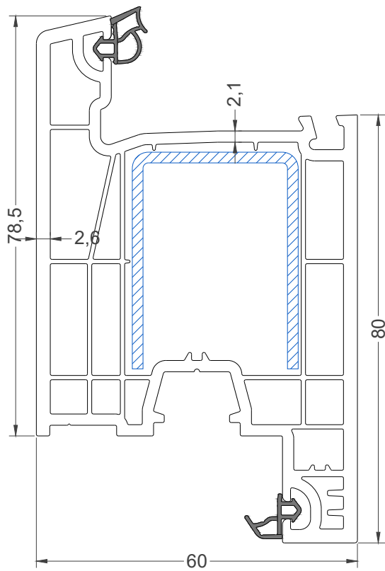
Дверная створка 78.5 мм (Z-type) Арт. 6104
