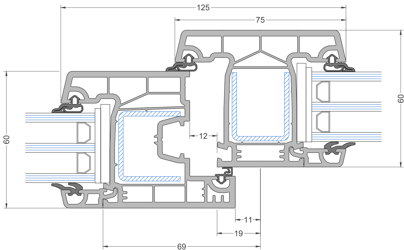
Арт. 6102 Створка
