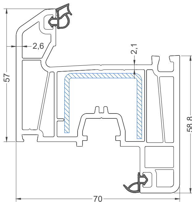
Створка 57 мм B-Class Арт. 7002
