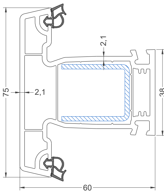
Импост 75 мм Арт. 6003
