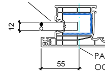
ОТВЕРСТИЕ ШПИНГАЛЕТА 12 мм
