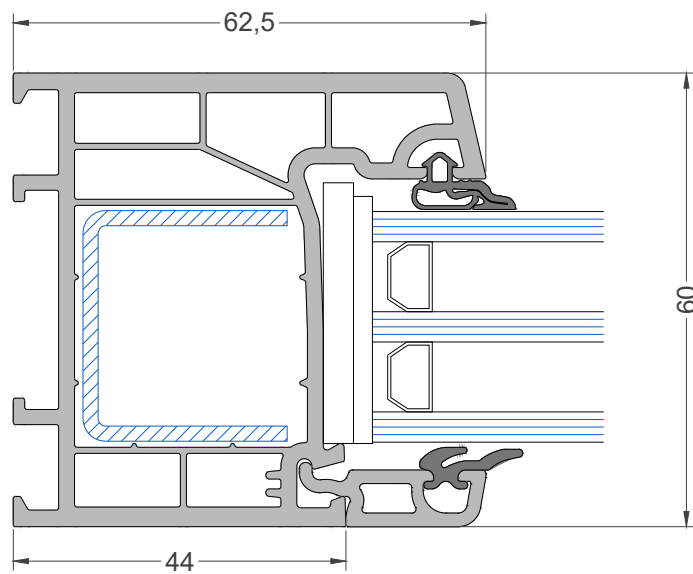
Арт. 6101 Рама
