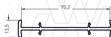
Артикул: 7011 Соединительная планка
