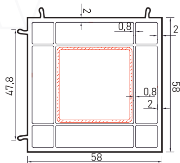
Артикул: 5806 Соед. профиль угловой 90°
