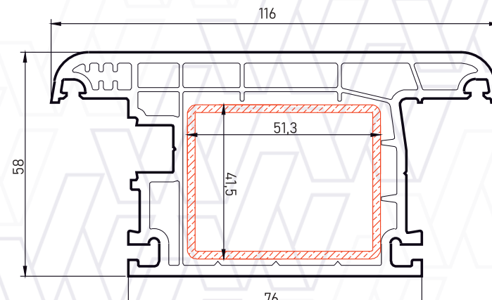
Артикул: 5805 Дверной профиль с внутренним открыванием
