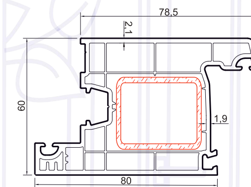
Дверной профиль с внутренним открыванием
