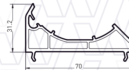
Артикул: 7007 Профиль адаптера к трубе
