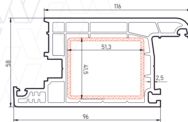
Артикул: 5804 Дверной профиль с наружным открыванием
