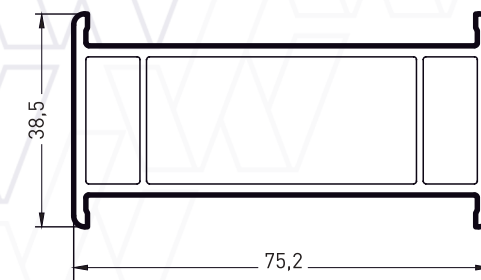
Артикул: 7010 Соединительный профиль
