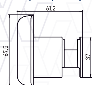
Артикул: 5812 Заглушка адаптера
