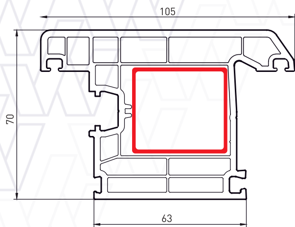
Артикул: 7005 Дверной профиль с наружным открыванием
