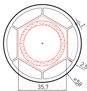
Артикул: 5809 Профиль трубы 58 мм
