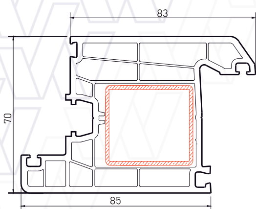
Артикул: 7004 Дверной профиль с внутренним открыванием
