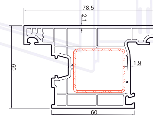
Дверной профиль с наружным открыванием
