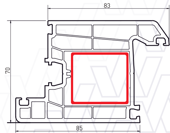
Артикул: 7004 Дверной профиль с внутренним открыванием
