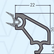
Артикул: 7014 Штапик 24 мм стекла
