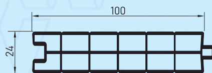
Артикул: 2401 Ламбри 24 мм
