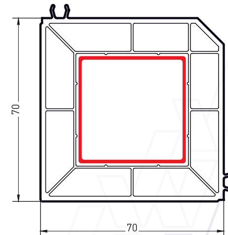
Артикул: 7008 Соединительный профиль угловой, 90°С
