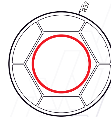
Артикул: 7006 Профиль трубы 70 мм
