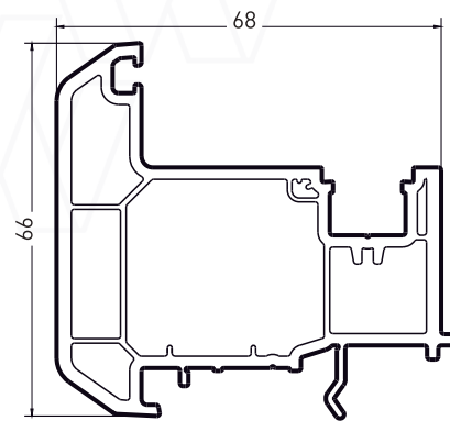
Артикул: 7009 Адаптер створки
