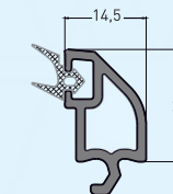
Артикул: 7013 Штапик 32 мм стекла
