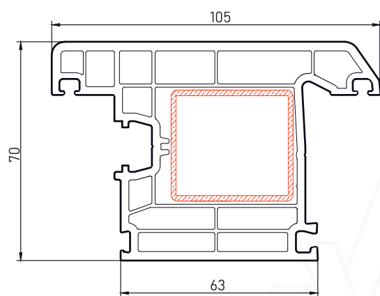
Артикул: 7005 Дверной профиль с наружным открыванием
