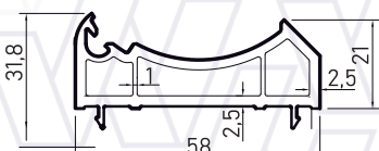
Артикул: 5810 Профиль адаптера трубы
