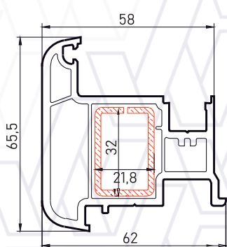
Артикул: 5811 Адаптер створки (штульп)
